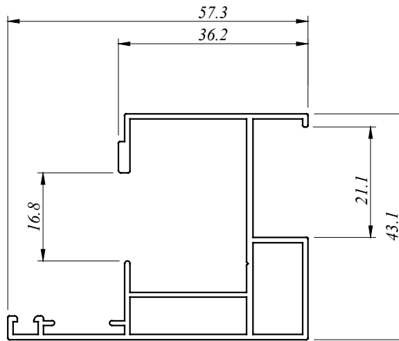
FUW 8901 0.656 Kg/M AP : 330.329 MM
