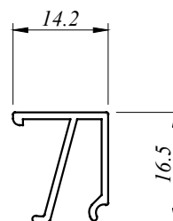
FUW 8903 0.656 Kg/M AP : 330.329 MM
