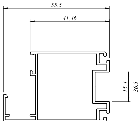
FUW 8902 0.655 Kg/M AP : 272.305 MM
