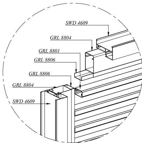
DETAILS A'
