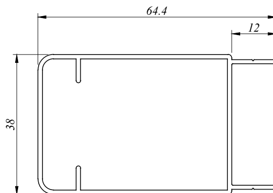
GRL 8804 0.693 Kg/M AP : 223.610 MM
