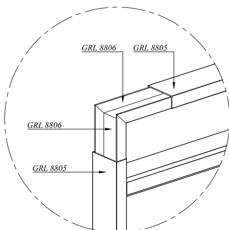
DETAILS A'
