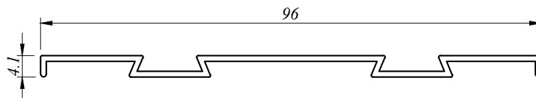
PT 7507 0.365 Kg/M AP : 238.665 MM
