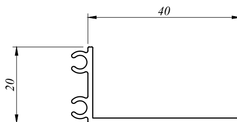
MISC 5141 0.268 Kg/M AP : 150.098 MM
