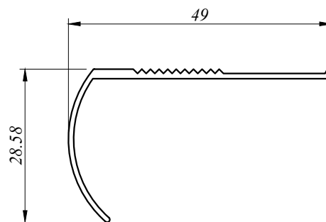
MISC 5103 0.244 Kg/M AP : 158.688 MM
