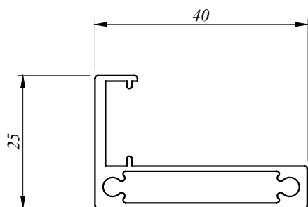
MISC 5138 0.450 Kg/M AP : 233.805 MM
