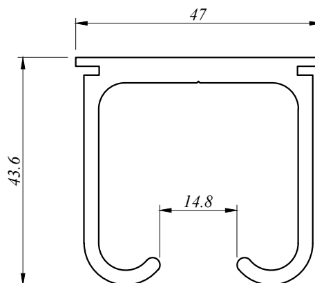
MISC 5126 1.327 Kg/M AP : 301.364 MM
