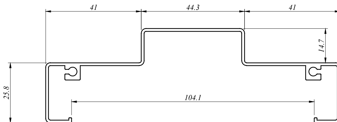
MISC 5145 H 0.891 Kg/M AP : 490.938 MM
