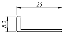
MISC 5114 0.124 Kg/M AP : 65.327 MM
