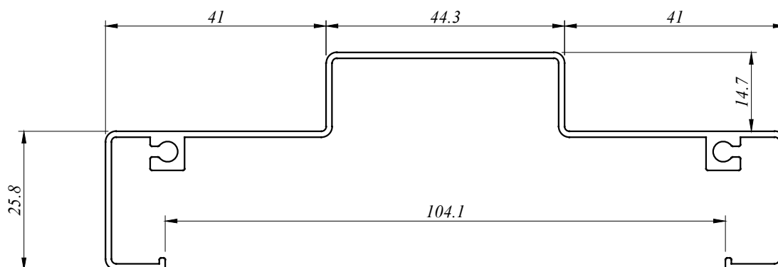
MISC 5145 0.801 Kg/M AP : 491.538 MM
