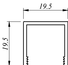
MISC 5119 0.218 Kg/M AP : 119.814 MM
