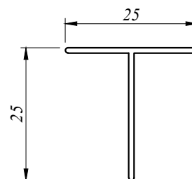
MISC 5118 0.140 Kg/M AP : 96.712 MM
