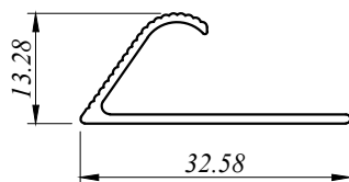
MISC 5102 0.178 Kg/M AP : 107.058 MM
