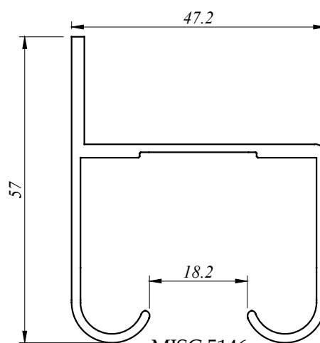
MISC 5146 0.825 Kg/M AP : 323.966 MM
