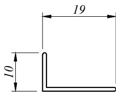
MISC 5121 0.075 Kg/M AP : 57.142 MM
