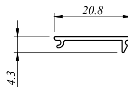
MISC 5137 0.070 Kg/M AP : 53.775 MM
