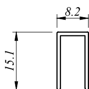
MISC 5125 0.089 Kg/M AP : 73.970 MM
