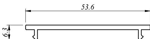
MISC 5144 0.316 Kg/M AP : 128.579 MM
