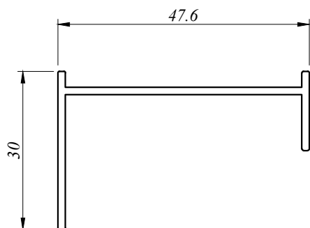
MISC 5142 0.340 Kg/M AP : 181.370 MM
