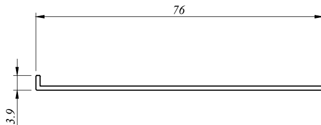
MISC 5122 0.235 Kg/M AP : 159.156 MM
