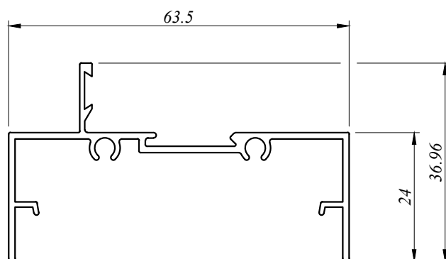
SWD 4606 0.570 Kg/M AP : 326.330 MM
