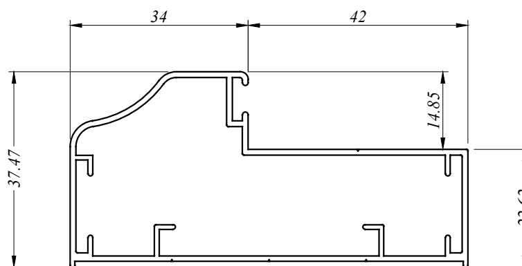
SWD 4611 0.750 Kg/M AP : 232.227 MM
