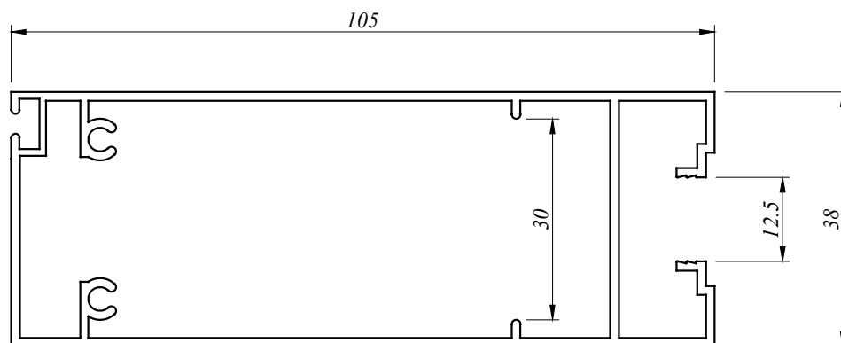
SWD 4608 1.292 Kg/M AP : 395.424 MM
