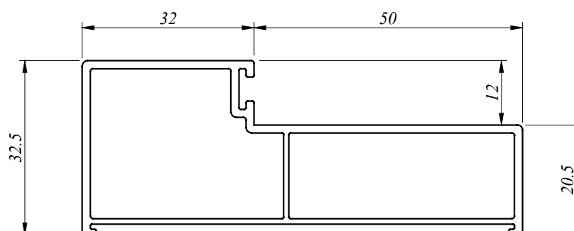
SWD 4612 0.897 Kg/M AP : 245.638 MM
