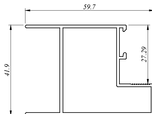
SWD 4602 0.841 Kg/M AP : 254.527 MM
