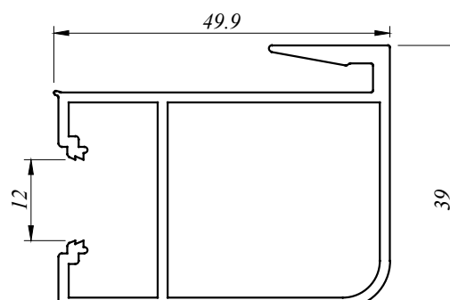
SD 4406 0.855 Kg/M AP : 277.732 MM
