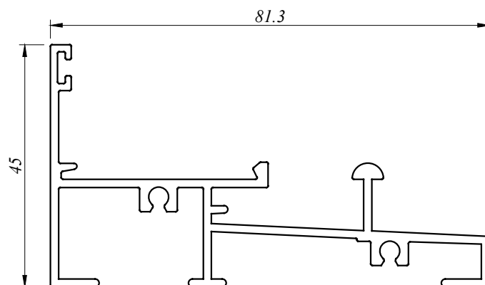
SD 4412 0.992 Kg/M AP : 460.169 MM
