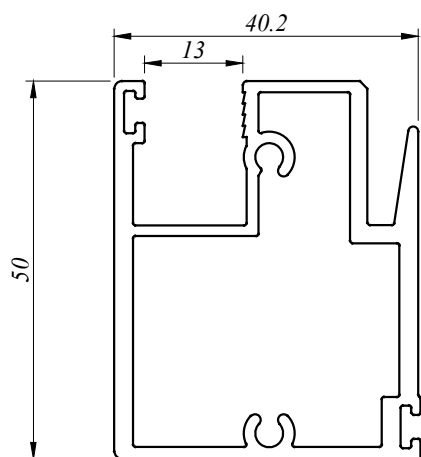
SD 4407 1.242 Kg/M AP : 263.831 MM
