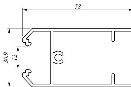
SD 4404 0.742 Kg/M AP : 361.897 MM
