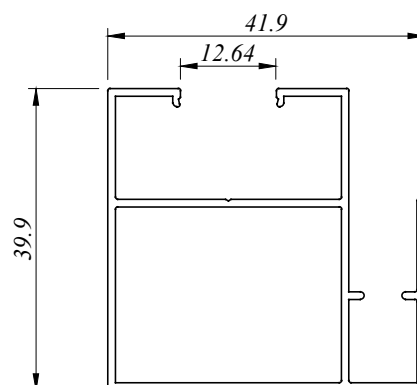
SD 4306 D 0.562 Kg/M AP : 287.073 MM
