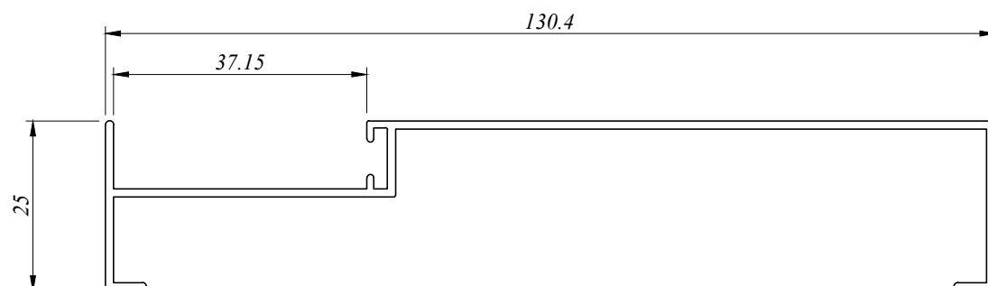
SD 4316 0.715 Kg/M AP : 408.424 MM
