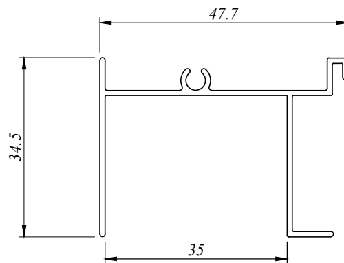
SD 4308 D 0.365 Kg/M AP : 266.122 MM
