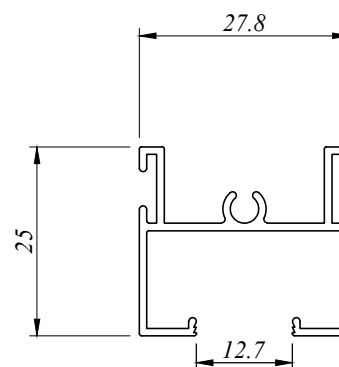
SD 4310 D 0.336 Kg/M AP : 225.789 MM
