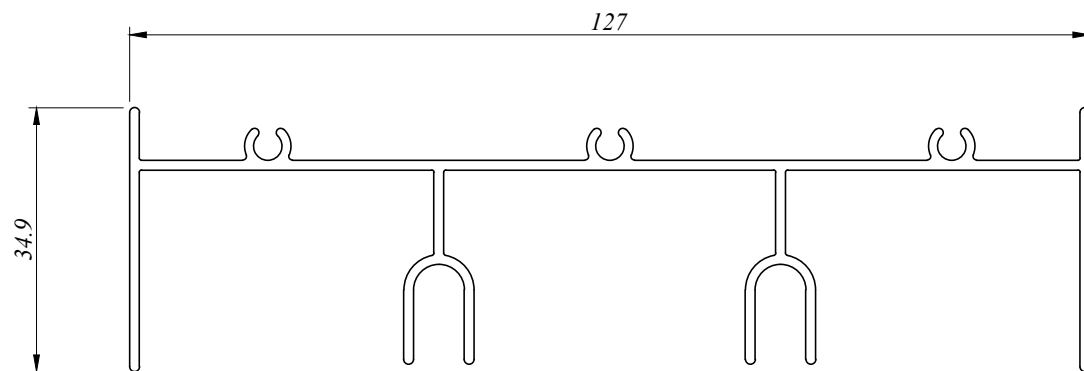
SD 4314 1.078 Kg/M AP : 608.395 MM
