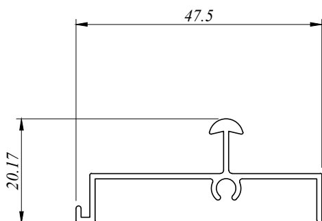
SD 4309 D 0.261 Kg/M AP : 176.759 MM
