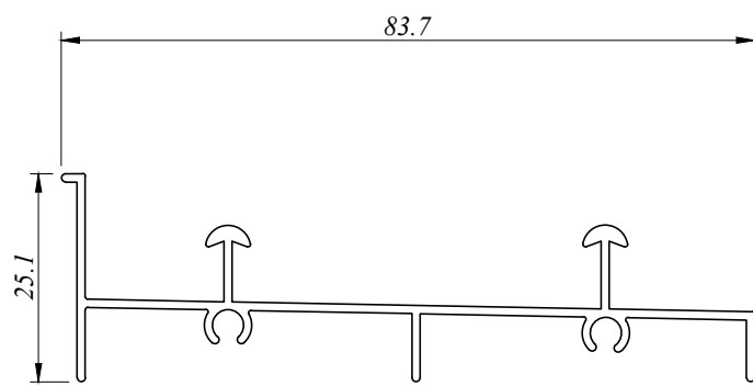
SD 4302 D 0.540 Kg/M AP : 331.680 MM
