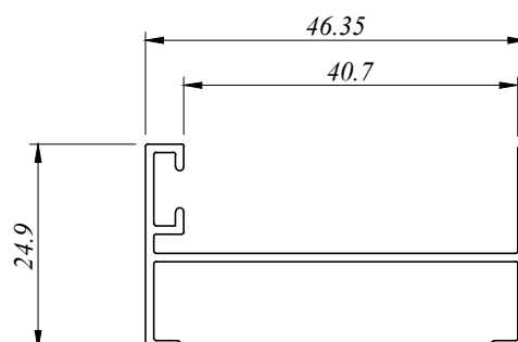
SD 4311 D 0.332 Kg/M AP : 223.438 MM
