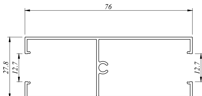
SD 4304 D 0.678 Kg/M AP : 433.779 MM
