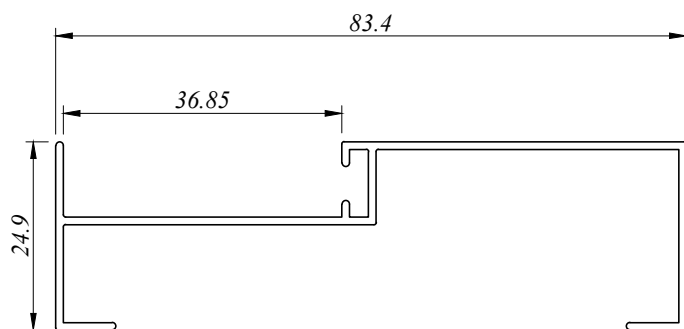
SD 4303 D 0.492 Kg/M AP : 330.295 MM
