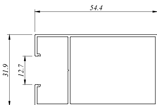
SD 4305 D 0.551 Kg/M AP : 241.251 MM
