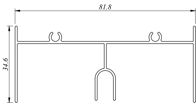
SD 4301 D 0.610 Kg/M AP : 414.759 MM
