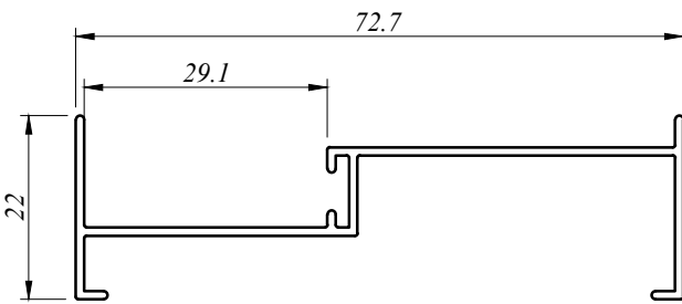
ESD 4203 D 0.382 Kg/M AP : 271.080 MM
