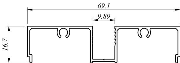
ESD 4212 D 0.451 Kg/M AP : 298.662 MM
