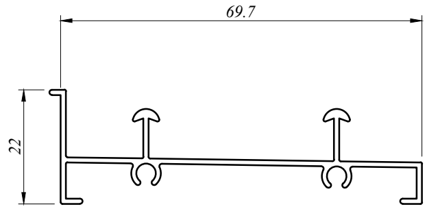
ESD 4202 D 0.450 Kg/M AP : 296.100 MM
