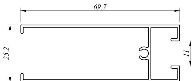
SD 4108 0.599 Kg/M AP : 387.783 MM
