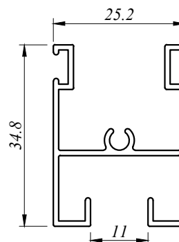
SD 4107 0.426 Kg/M AP : 268.880 MM
