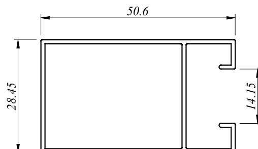
SD 4109 0.528 Kg/M AP : 226.069 MM
