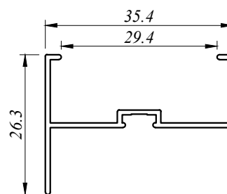
SD 4111 0.249 Kg/M AP : 192.067 MM
