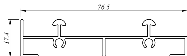
SD 4106 0.630 Kg/M AP : 325.355 MM
