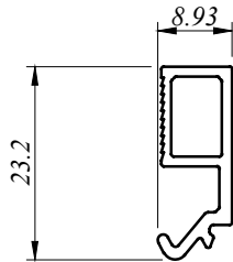
ACW 3847 0.199 Kg/M AP : 79.908 MM
