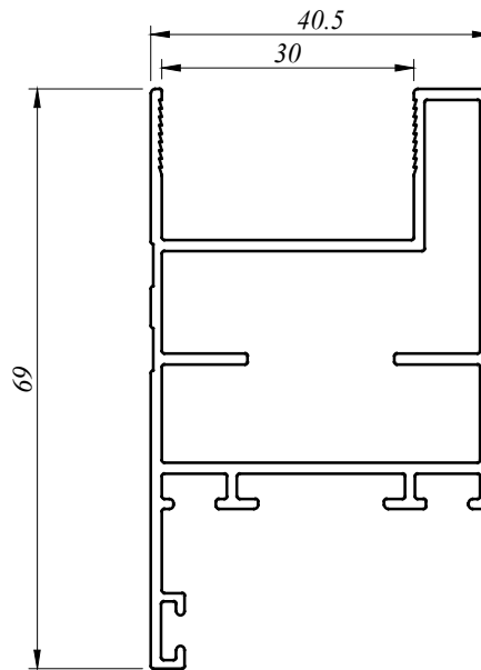
ACW 3849 0.906 Kg/M AP : 318.980 MM
