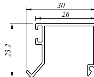
ACW 3833 0.225 Kg/M AP : 166.045 MM
