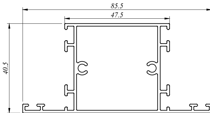
ACW 3832 0.933 Kg/M AP : 372.782 MM
