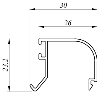
ACW 3836 0.214 Kg/M AP : 158.148 MM
