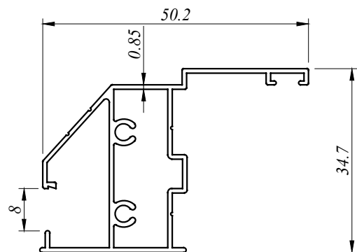
CW 3380 B 0.445 Kg/M AP : 363.92 MM
