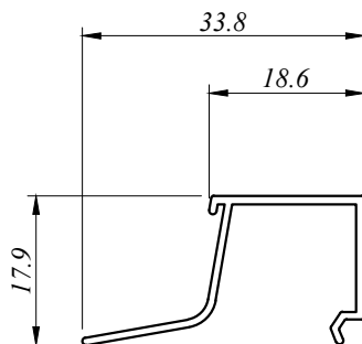
CW 3302 D 0.184 Kg/M AP : 135.450 MM
