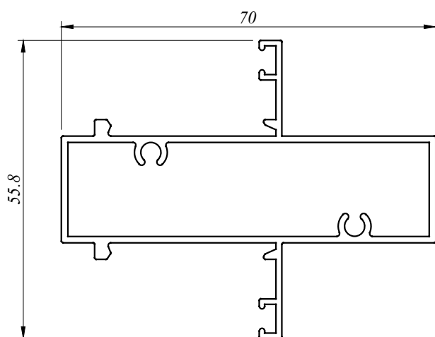
CW 3313 H 0.903 Kg/M AP : 500.810 MM
