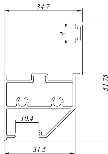
CW 3382 D 0.505 Kg/M AP : 245.478 MM
