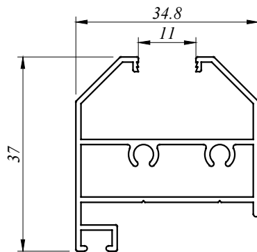
CW 3307 D 0.540 Kg/M AP : 236.530 MM
