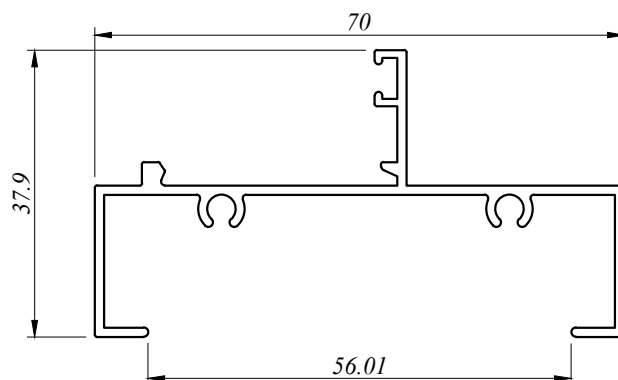
CW 3312 H 0.588 Kg/M AP : 329.898 MM
