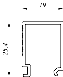
CW 3352 D 0.215 Kg/M AP : 152.560 MM
