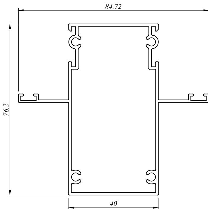
CW 3377 H 1.070 Kg/M AP : 368.470 MM
