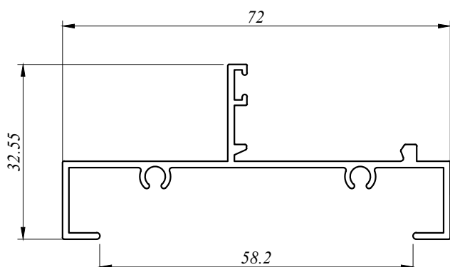
CW 3311 H 0.561 Kg/M AP : 321.900 MM
