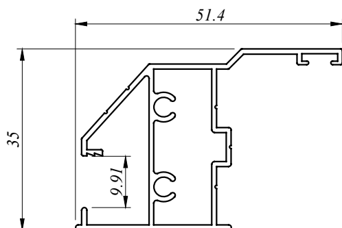
CW 3367 D 0.505 Kg/M AP : 245.960 MM
