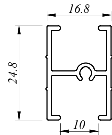
CW 3355 D 0.220 Kg/M AP : 158.452 MM
