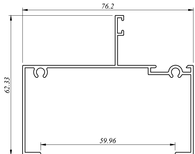
CW 3378 F 0.661 Kg/M AP : 438.362 MM
