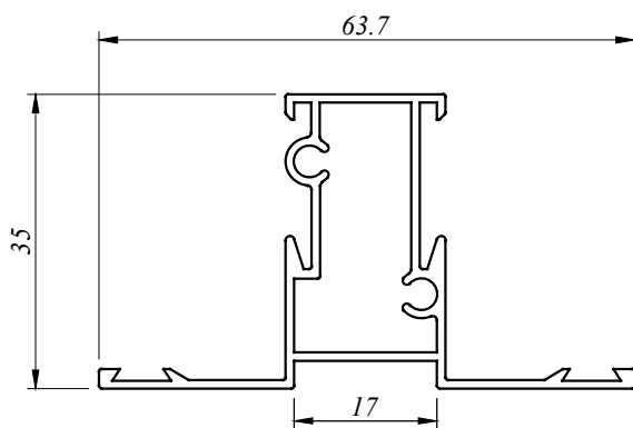
CW 3379 D 0.538 Kg/M AP : 252.911 MM
