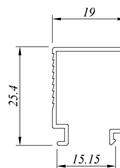
CW 3384 0.215 Kg/M AP : 155.87 MM
