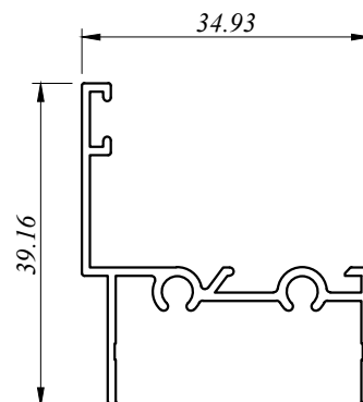
CW 3369 D 0.346 Kg/M AP : 231.377 MM
