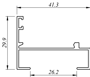
CW 3301 D 0.318 Kg/M AP : 209.062 MM
