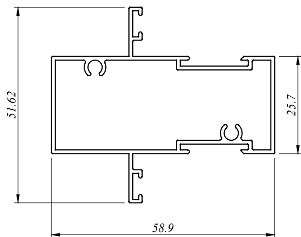
CW 3364 D 0.776 Kg/M AP : 261.090 MM
