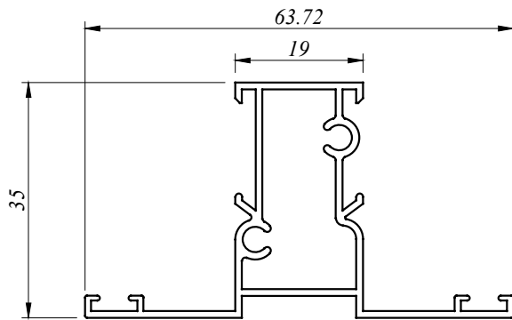
CW 3370 D 0.553 Kg/M AP : 265.848 MM
