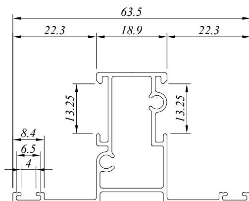
CW 3383 D 0.553 Kg/M AP : 259.166 MM
