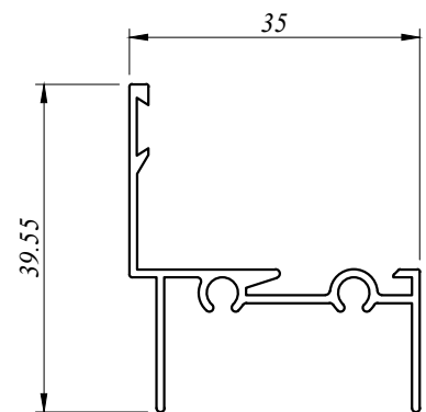
CW 3376 0.326 Kg/M AP : 225.521 MM
