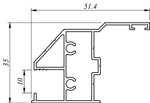
CW 3373 D 0.527 Kg/M AP : 219.870 MM
