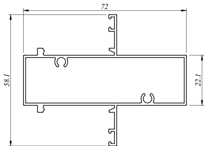
CW 3310 H 0.896 Kg/M AP : 305.000 MM
