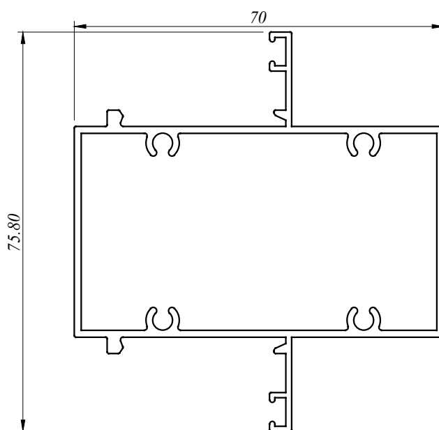
CW 3314 J 1.158 Kg/M AP : 340.049 MM
