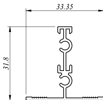
CW 3359 D 0.299 Kg/M AP : 198.240 MM
