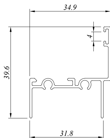
CW 3381 D 0.346 Kg/M AP : 229.428 MM
