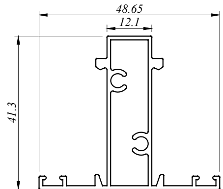
CW 3304 D 0.560 Kg/M AP : 226.114 MM
