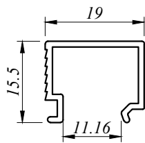
CW 3351 0.140 Kg/M AP : 113.180 MM
