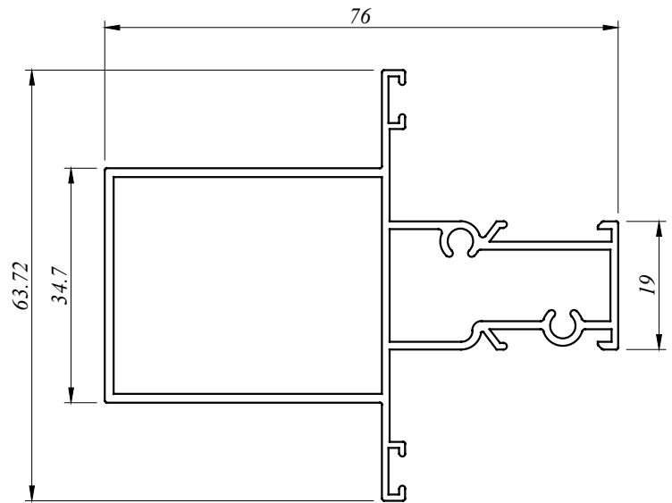
CW 3372 1.002 Kg/M AP : 339.749 MM
