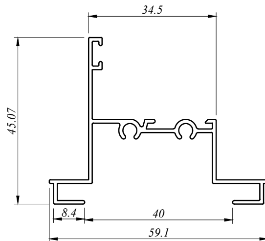
CW 3207 0.498 Kg/M AP : 330.070 MM
