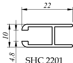
SHC 2201 0.189 Kg/M AP : 108.230 MM
