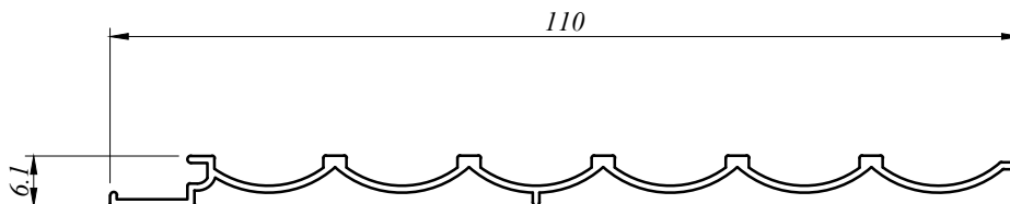
SHC 2208 0.338 Kg/M AP : 266.127 MM
