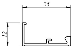
SHC 2205 0.138 Kg/M AP : 90.551 MM
