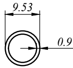
RT 140309 0.066 Kg/M AP : 29.939 MM
