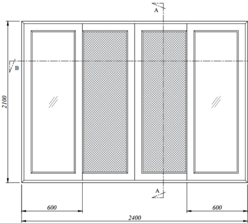
M SLIDNG DOOR
