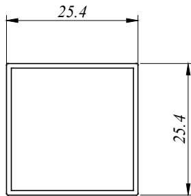
SH 25080810 0.272 Kg/M AP : 101.085 MM
